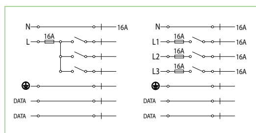
Fig. 3 Schema elettrico Pic. 3 Electrical scheme
