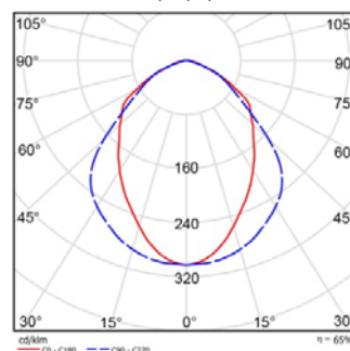
DISPLAY 51150/W/1/E
